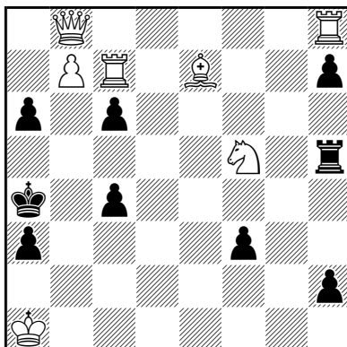
524 + (7+9)
