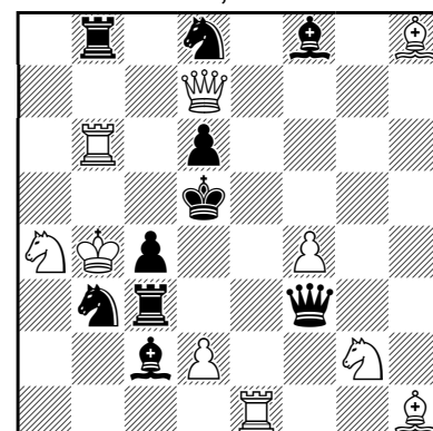
504 #2 (10+10)
