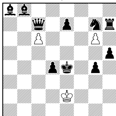
521 h#3 (3+10) 2.1.1.1.1.1
