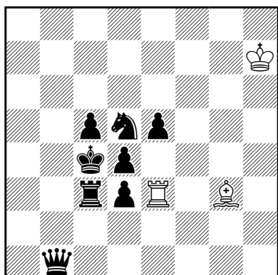
520 h#3 (3+8) 2.1.1.1.1.1
