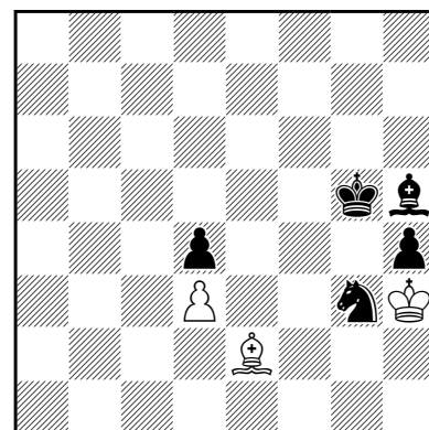
465 h#5 (3+5)
