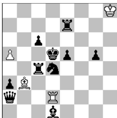
h # 3 b)Rd1→f1 (4 + 10)
