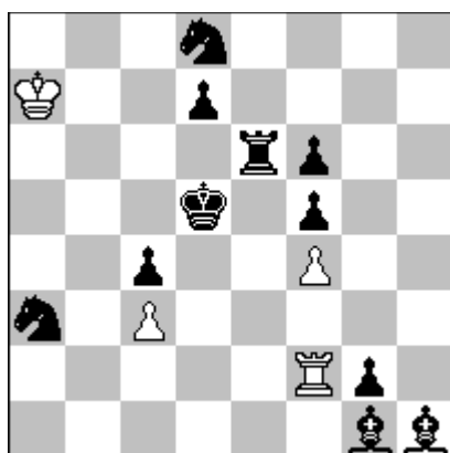
h # 3 2.1.1.1.1.1 (4 + 11)
