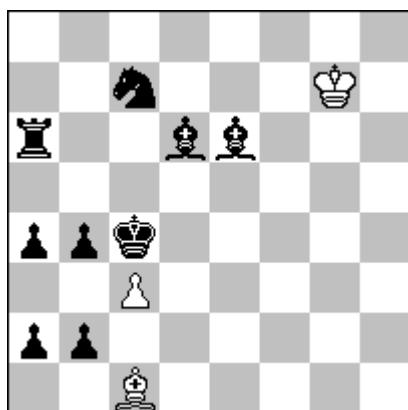
h # 3 2.1.1.1.1.1 (3 + 9)
