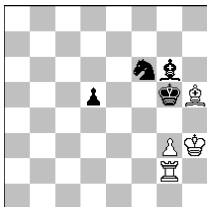
h # 3 2.1.1.1.1.1 (4 + 4)
