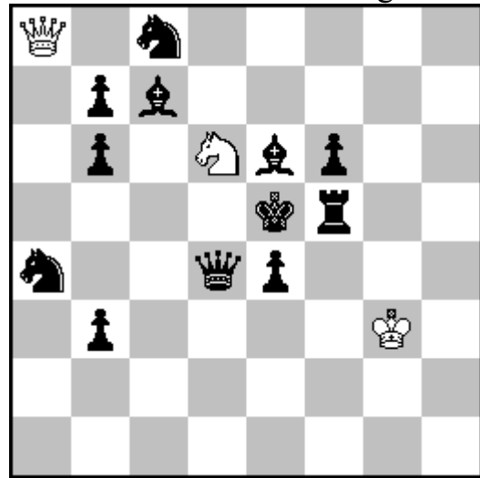
h#2 2 Lösungen 3+12
