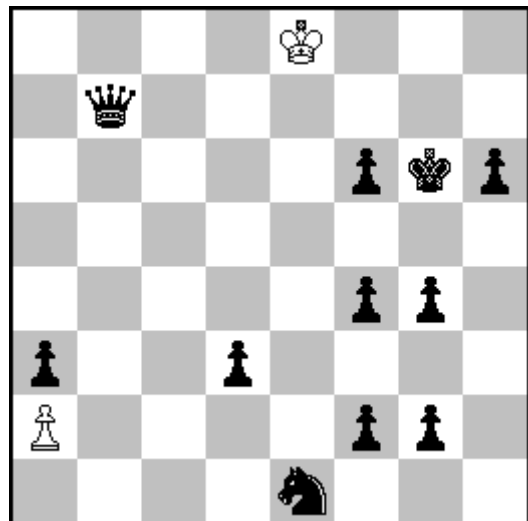
h#7 2+11
