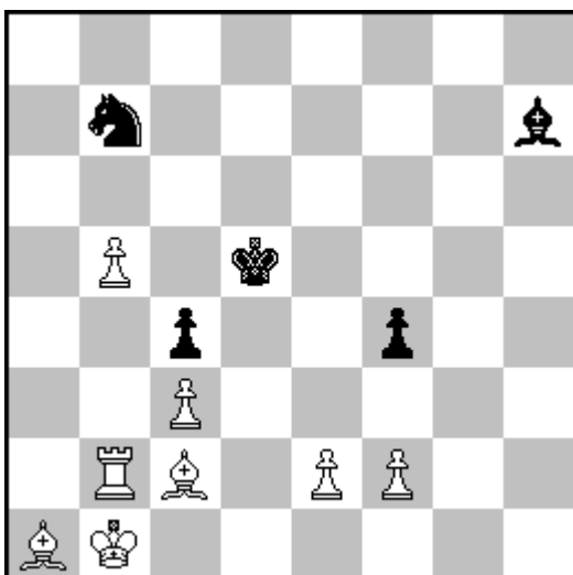
h#3 2 Lösungen 8+5
